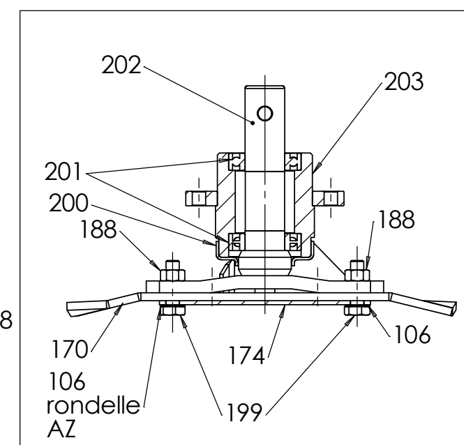
A-A (1 : 4)
