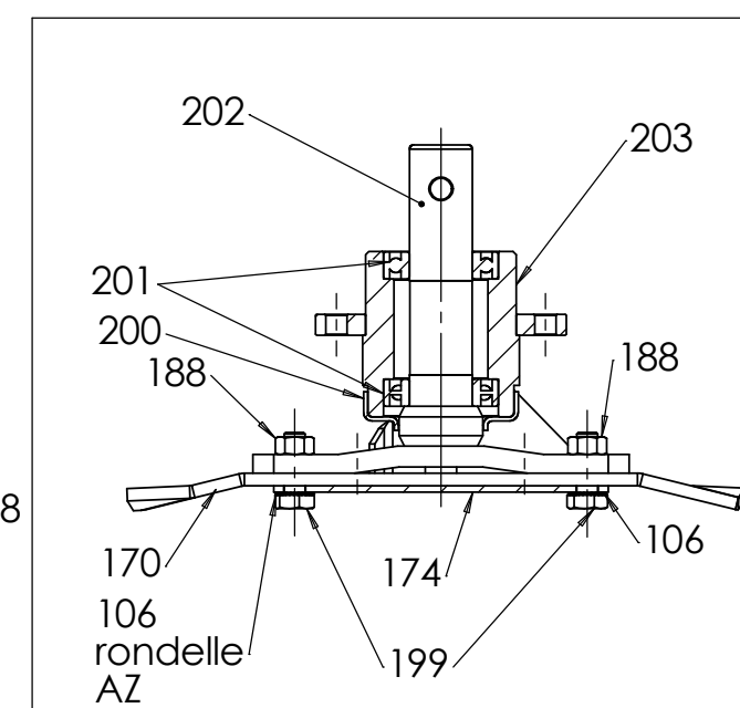
A-A (1 : 4)
