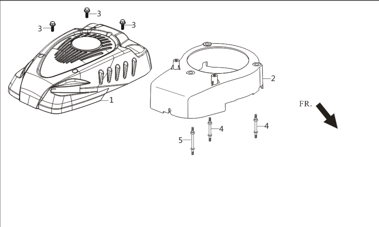
FIG.7 SHIELD, FAN (E07)
