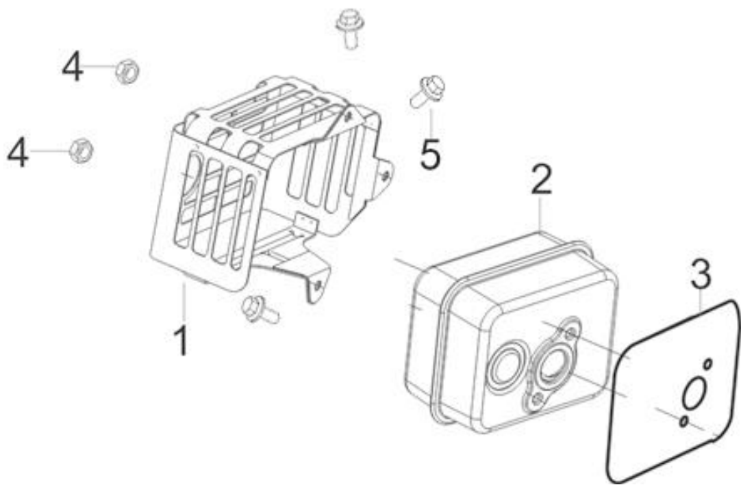
FIG.10 MUFFLER (E10)
