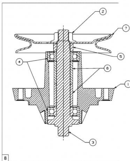
Spindle Assembly / Messerwelle 618-04474
