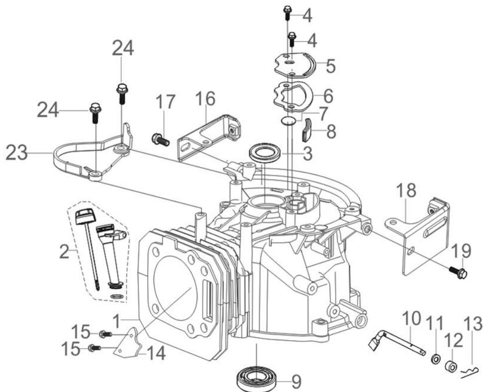
FIG.2 CRANKCASE. (E02)
