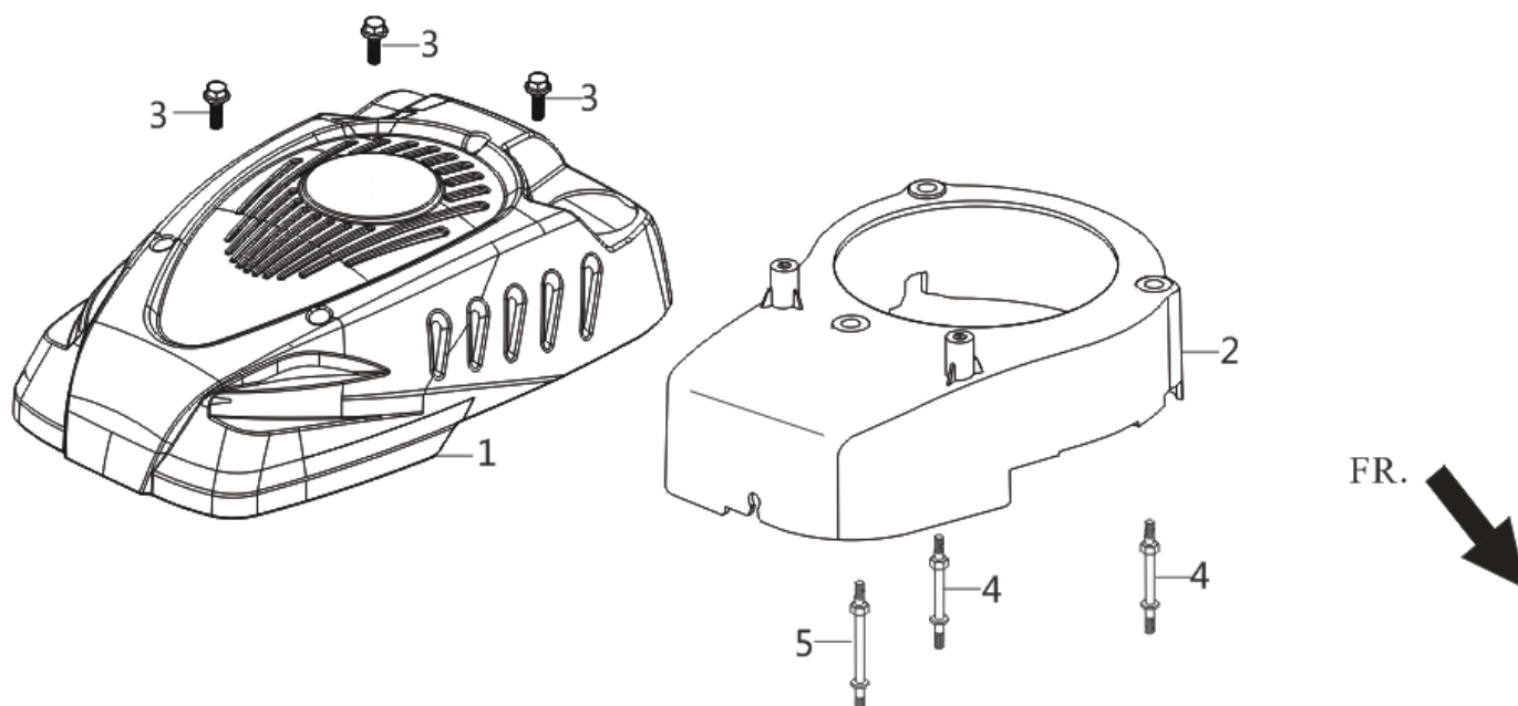
FIG.7 SHIELD, FAN (E07)
