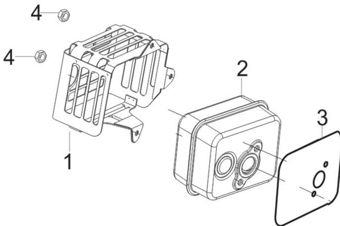
FIG.10 MUFFLER (E10)
