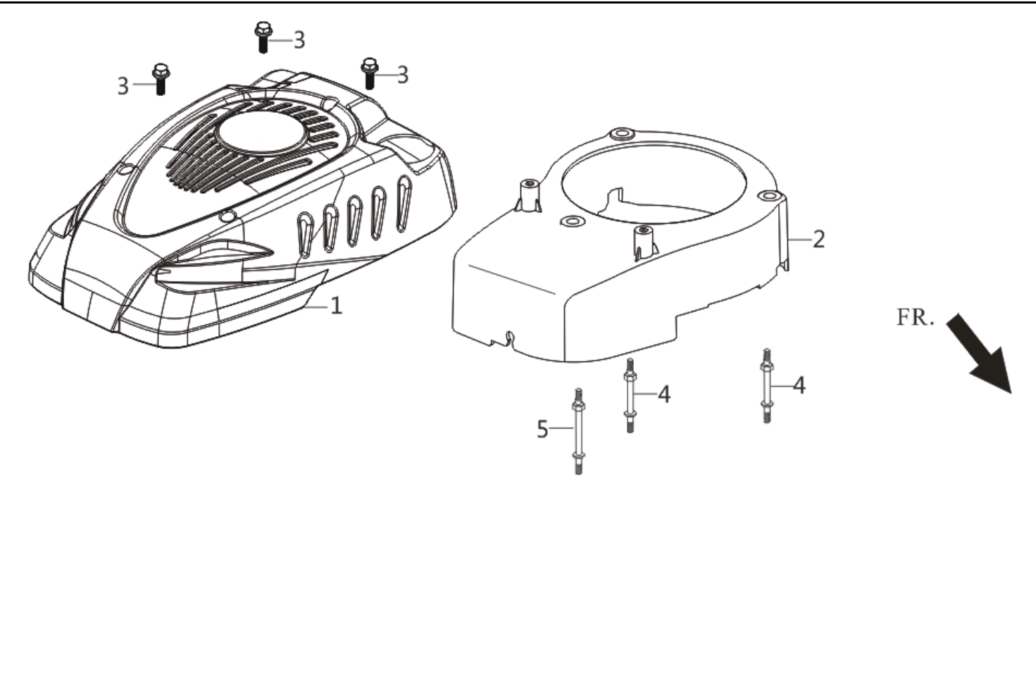
FIG.7 SHIELD, FAN (E07)
