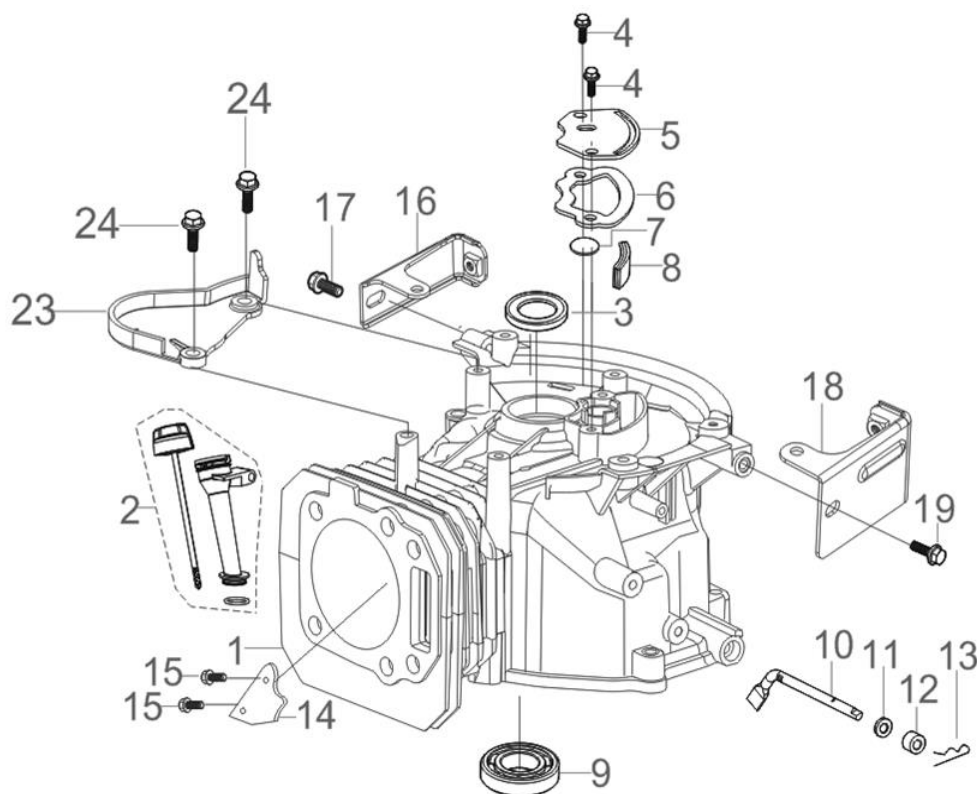
FIG.2 CRANKCASE. (E02)
