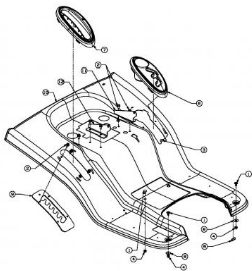
E3-02040A-01
