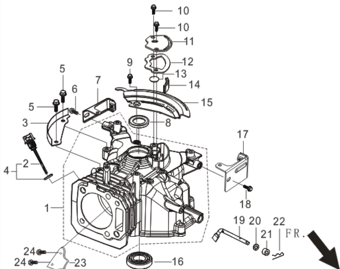
FIG.1 CRANKCASE. (E01)
