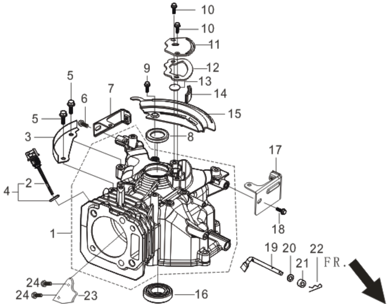
FIG.1 CRANKCASE. (E01)
