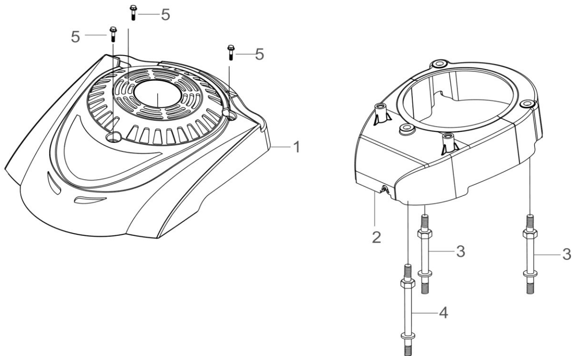
FIG.7 SHIELD, FAN (E07)
