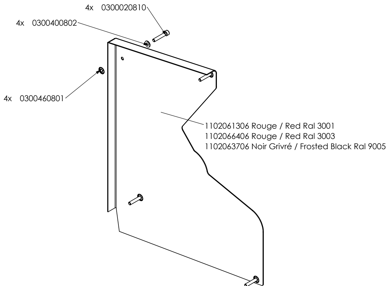
11_Capot Lampe Mobile Ø505_Défaut
