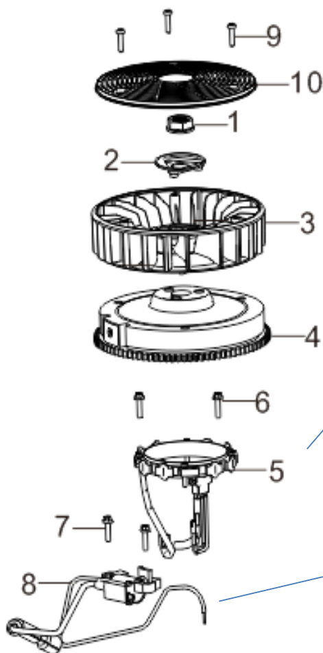
FIG.10 VOLANT MOTEUR - FLYWHEEL (E10)
