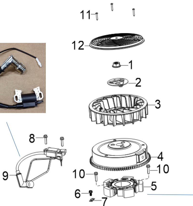
FIG.10 VOLANT MOTEUR - FLYWHEEL (E10)
