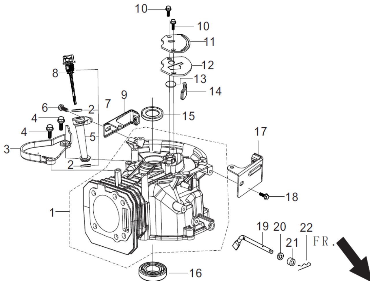
FIG.2 CRANKCASE. (E01)
