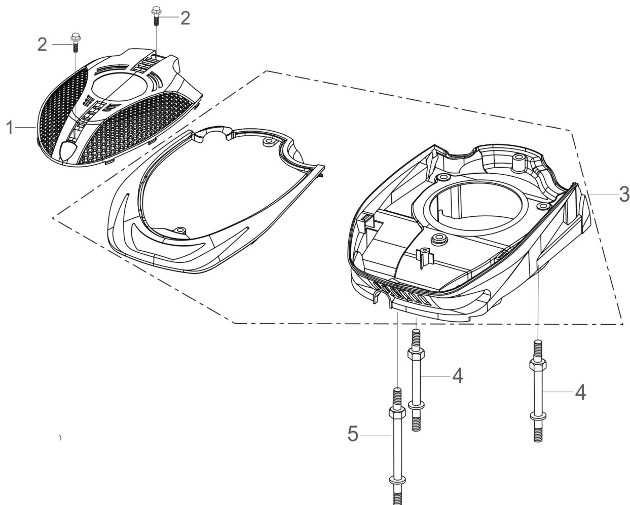
FIG.7 SHIELD, FAN (E14)
